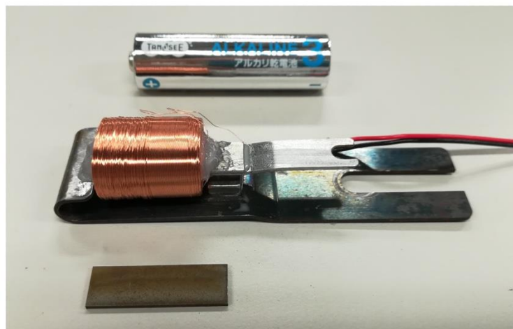
写真 2:振動発電デバイス(中)と、これに利用している幅 8mm×厚さ 1mm×長さ 26mm の Fe-Ga 単結晶合金の板(下)と単 3 乾電池(上)。デバイスは 20~100Hz の振動でミリワットの電力を出力する。半永久の寿命を持ち、IoT(無線通信センサモジュール)の電池(通常、長くて3年で交換)を代替する。従来、この単結晶板が高価なことが商品化における課題であった。今回の技術革新により、上述の単結晶板の数百円/枚での生産が現実となり、磁歪振動発電デバイスが大幅に安価になることで、電池フリーモジュール・システムを用いた各分野で IoT の実用化が加速されると確信する。
